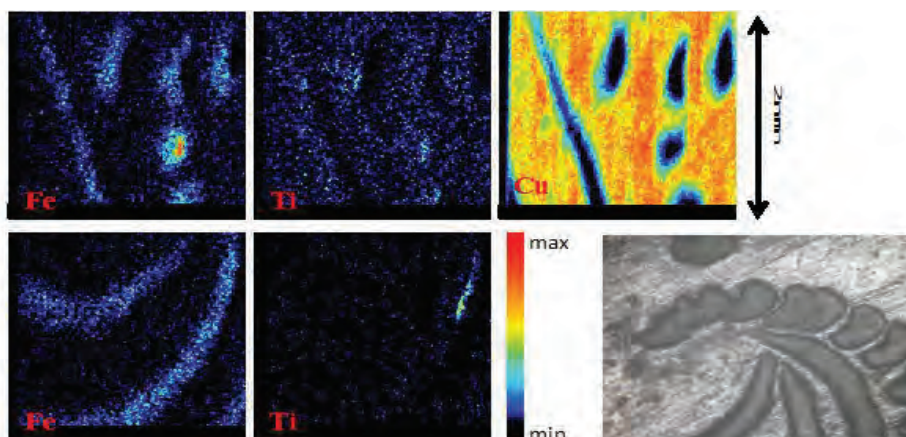
16. b kép: A pásztázó mikroszkóppal felvett elemtérképek a hajdúsámsoni kard díszítésén, valamint mikroszkóppal (Nikon sztereo) készített felvétel az egyik motívumon. Jól látható az inhomogenitás a különböző motívumokban.
