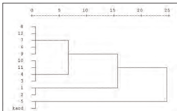
14. kép: A hajdúsámsoni kincs PIXE eredményein végzett klaszteranalízis során kapott dendrogram.
