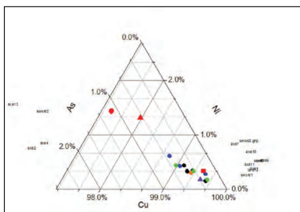
15. kép: Ternary diagram a hajdúsámsoni és a téglási kincsek Cu, Ni és As wt% tartalmának figyelembe vételével. A piros kör a téglási csákány, a háromszög a téglási kard pengéje, a négyzet pedig a markolata.
