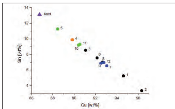
13. kép: A hajdúsámsoni leletek két fő összetevőjének százalékos aránya. Különböző színnel a megfelelő tipológiai csoportok: zöld – nyakkorongos csákány; fekete – nyéllyukas csákány; kék – dudoros nyéllyukas csákány; narancs – nyélcsöves csákány (ún. Křtěnov-típus).
