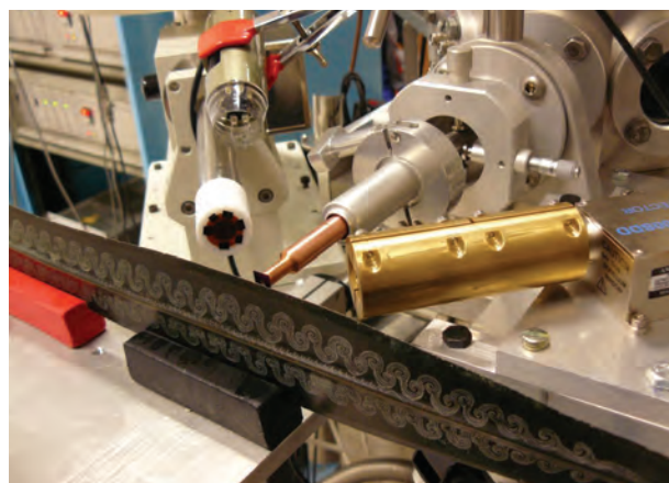
12. kép: A hajdúsámsoni presztízskard vizsgálata az Atomki nukleáris pásztázó mikroszondájának kihozott nyalábos elrendezésével. A fókuszált ionnyaláb egy vékony Si 3 N 4 fólián lép ki a levegőre. A keletkezett röntgen fotonokat két detektor (hagyományos Si(Li) és SDD) érzékeli a kilépő csőrvég két oldalán. Az SDD detektort egy mágnes védi a szórt protonoktól.
